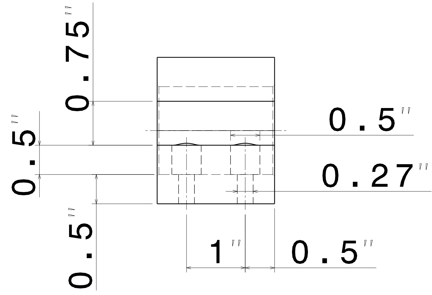
Right view Scale: 1:1
