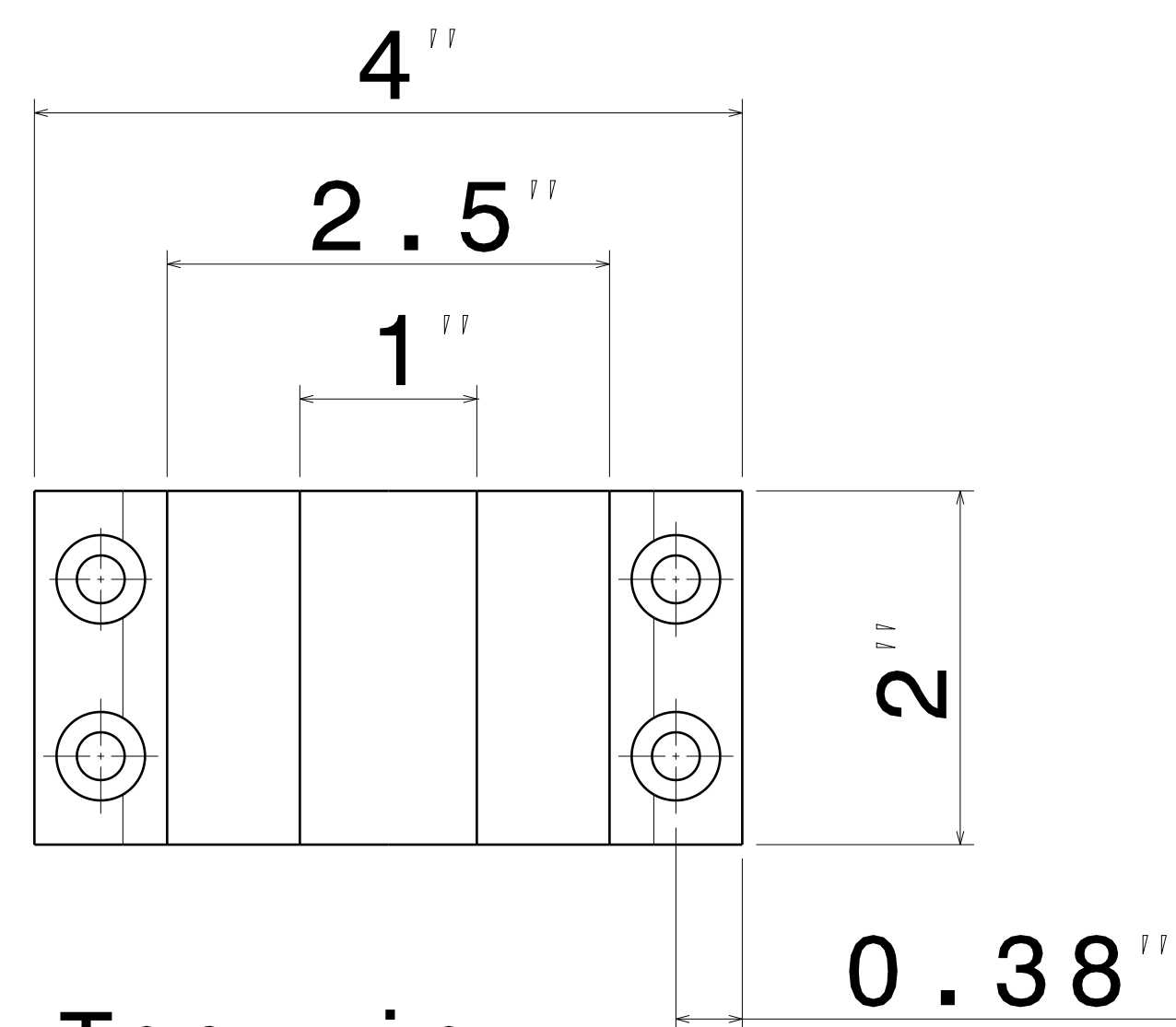
Top view Scale: 1:1
