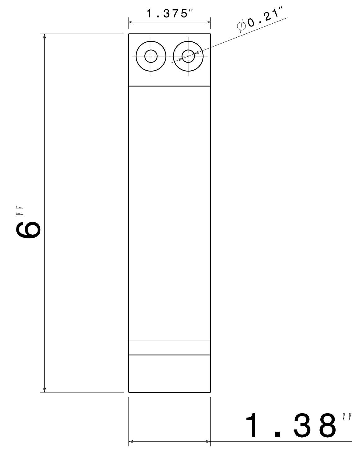
Right view Scale: 1:1
